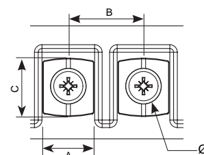
Borne M5
