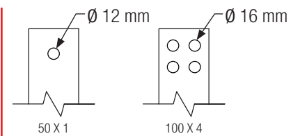
Conexión pletina
