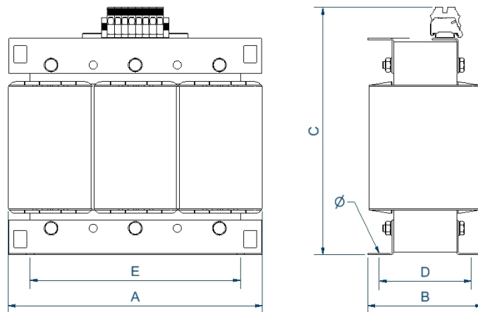
Dimensions (AxBxCxDxE): 180x84x203x66x150 mm 6Ø
