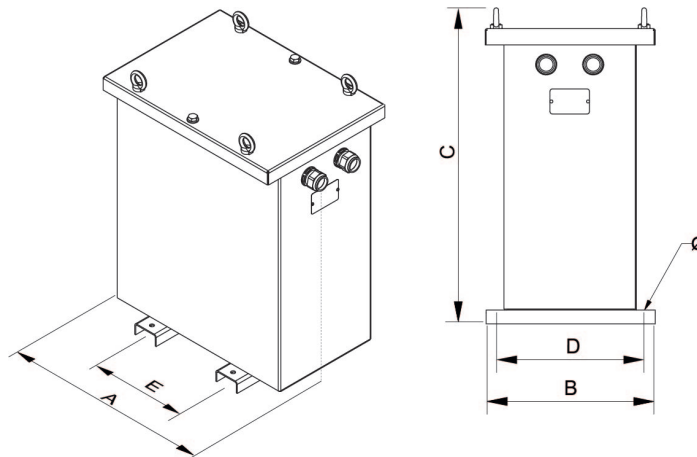
Dimensions (AxBxCxDxE): 330x284x463x230x200 mm 11Ø
