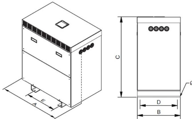
Dimensiones (AxBxCxDxE): 1200x760x1555x672x690 mm 18º
