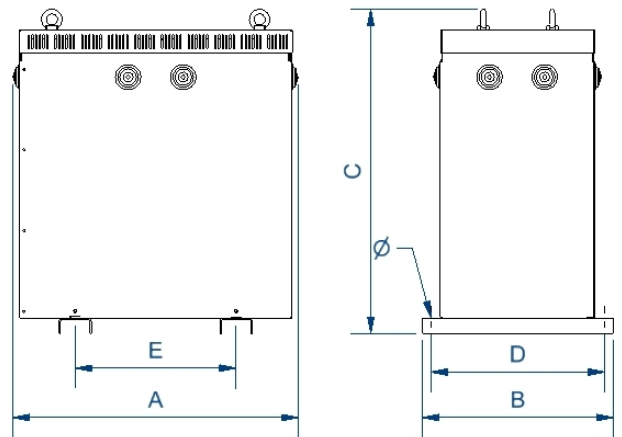
Dimensions (AxBxCxDxE): 315x230x315x205x200 mm 6Ø
