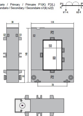
Dimensiones (AxBxCxDxE): 114x50x145 mm
