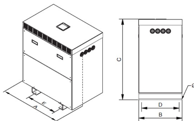
Dimensiones (AxBxCxDxE): 795x550x970x500x415 mm 12°
