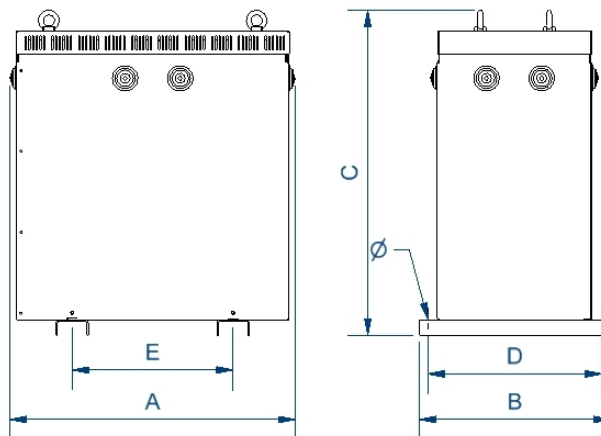
Dimensions (AxBxCxDxE): 315x230x315x205x200 mm 6Ø
