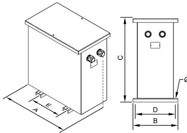
Dimensions (AxBxCxDxE): 350x284x463x230x200 mm 11Ø
