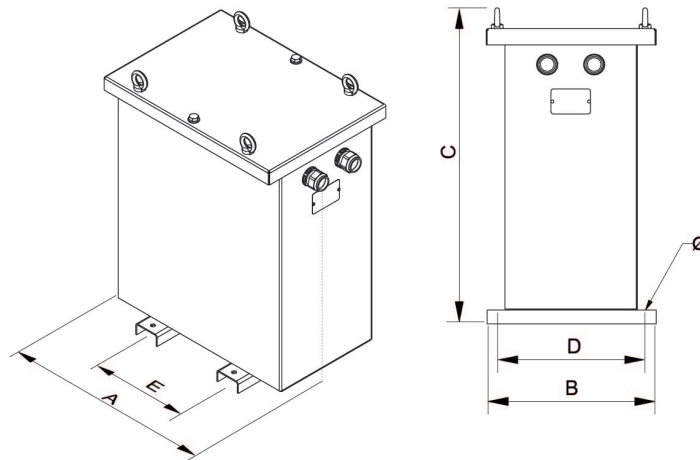
Dimensions (AxBxCxDxE): 350x284x463x230x200 mm 11Ø
