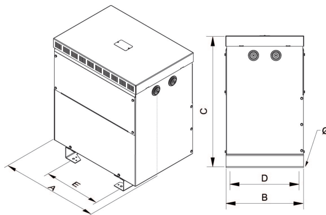
Dimensiones (AxBxCxDxE): 597x415x710x375x345 mm 12
