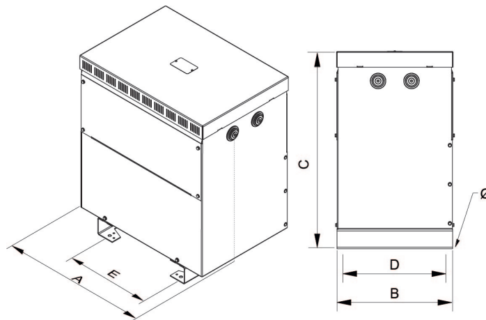
Dimensiones (AxBxCxDxE): 597x415x710x375x345 mm 12
