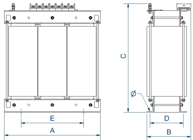
Dimensiones (Ax BxCxDxE): 670x300x615x190x426 mm 13
