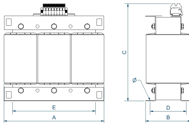
Dimensiones (AxBxCxDxE): 670x280x615x170x426 mm 13°
