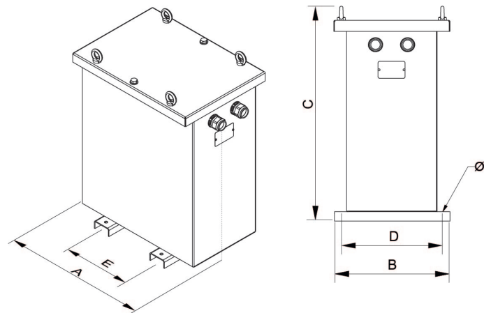
Dimensiones (AxBxCxDxE): 510x362x689x320x250 mm 11
