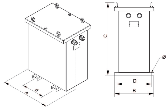
Dimensiones (Ax BxCxDxE): 694x413x764x370x350 mm 11
