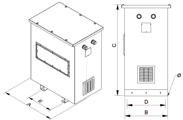
Dimensiones (AxBxCxDxE): 1050x900x1370x714x485 mm 18Ø
