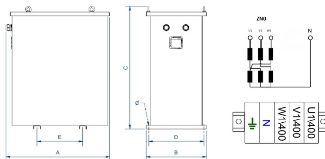
Dimensiones (AxBxCxDxE): 694x413x764x370x350 mm 11Ø
