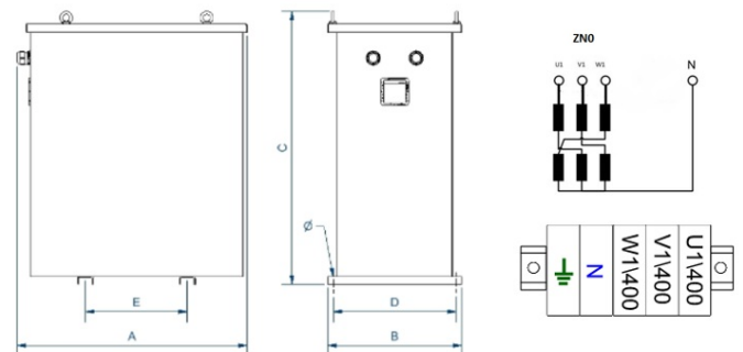
Dimensiones (AxBxCxDxE): 510x362x689x320x250 mm 11Ø
