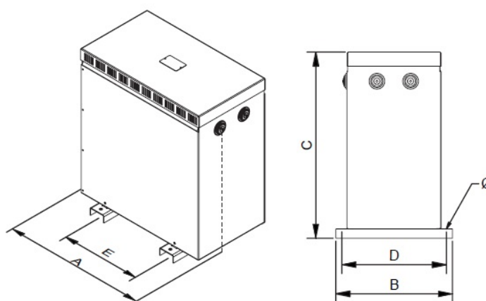
Dimensions (AxBxCxDxE): 310x230x308x205x197 mm 6Ø
