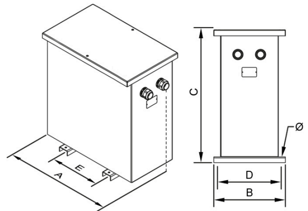
Dimensiones (AxBxCxDxE): 330x284x463x230x200 mm 11Ø
