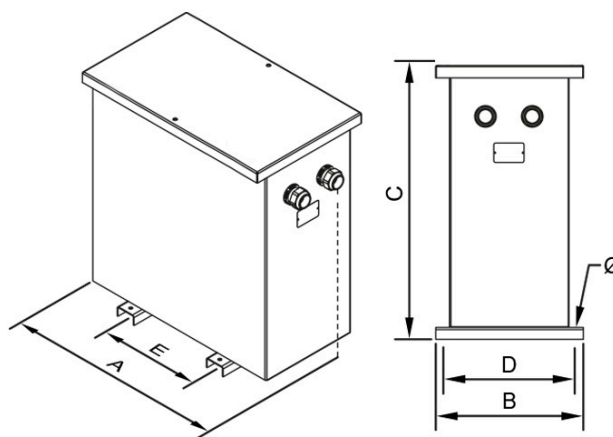
Dimensions (AxBxCxDxE): 330x284x463x230x200 mm 11Ø
