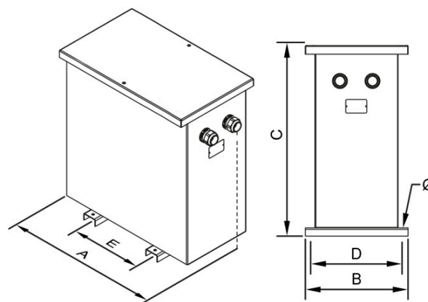
Dimensiones (AxBxCxDxE): 330x284x463x230x200 mm 11Ø
