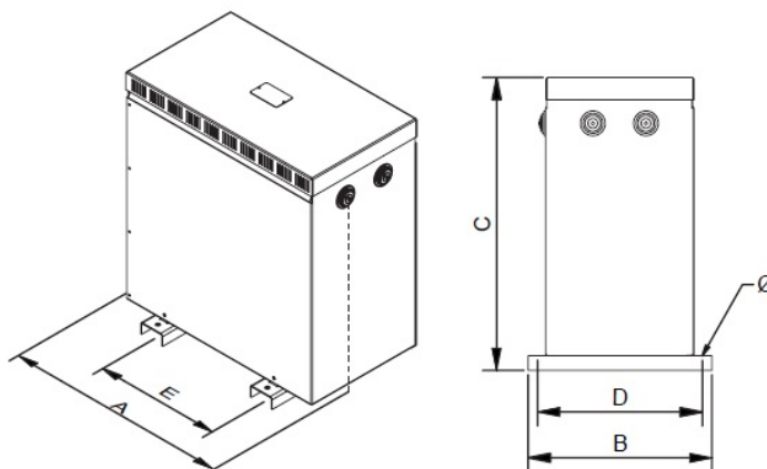
Dimensiones (AxBxCxDxE): 385x260x384x245x250 mm 6Ø
