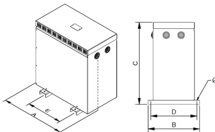
Dimensiones (AxBxCxDxE): 240x190x250x180x150 mm 6Ø
