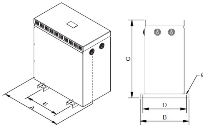
Dimensiones (AxBxCxDxE): 597x415x710x375x350 mm 12∅
