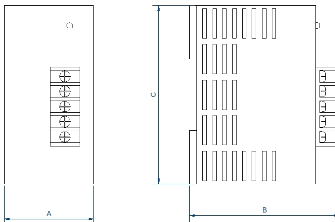
Dimensiones (AxBxCxDxE): 56x121x110 mm
