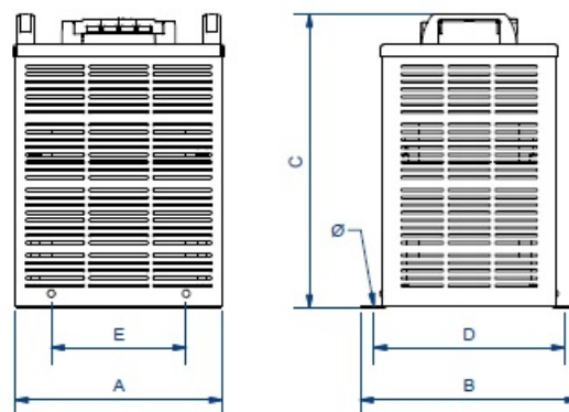
Dimensiones (AxBxCxDxE): 252x260x349x233x223 mm 70
