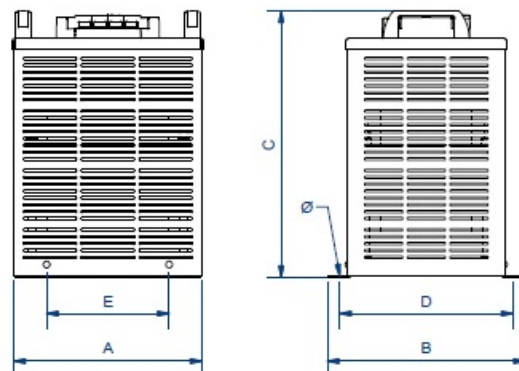
Dimensiones (AxBxCxDxE): 252x260x349x233x223 mm 7Ø
