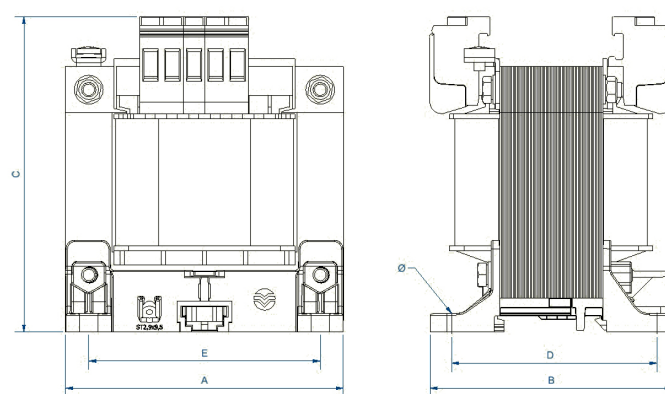
Dimensions (AxBxCxDxE): 75x82x89,5x71x62,5 mm 6
