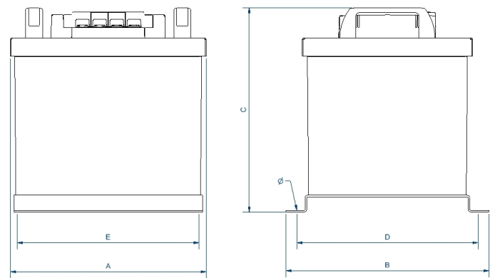
Dimensiones (AxBxCxDxE): 233x241x244x219x175 mm 7Ø
