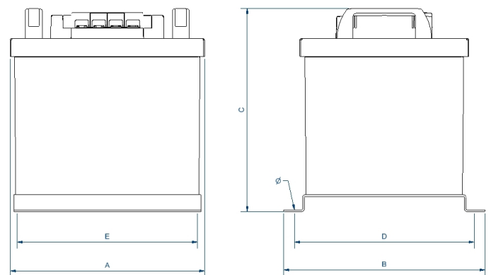
Dimensiones (AxBxCxDxE): 233x241x274x219x175 mm 7∅
