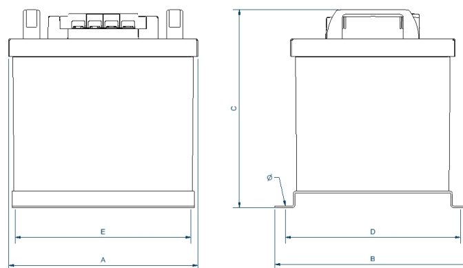
Dimensiones (AxBxCxDxE): 233x241x314x219x175 mm 7∅
