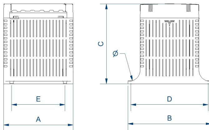
Dimensiones (AxBxCxDxE): 84x101x98x89x55 mm \varnothing
