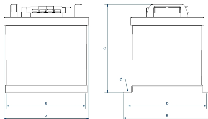
Dimensiones (AxBxCxDxE): 233x241x274x219x175 mm 7Ø
