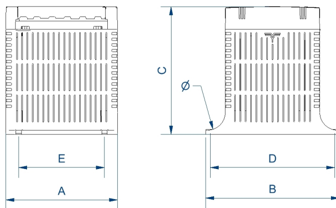
Dimensiones (AxBxCxDxE): 69x92x80x79x45 mm 5Ø
