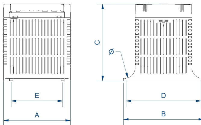
Dimensiones (AxBxCxDxE): 118x138x132x122x88 mm 5∅
