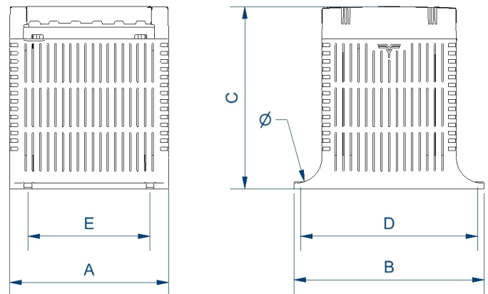
Dimensiones (AxBxCxDxE): 136x162x180x146x104 mm 6Ø
