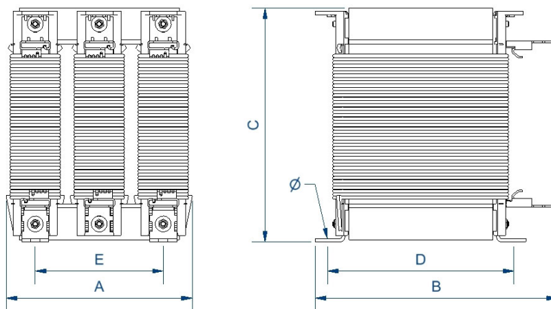
Dimensiones (AxBxCxDxE): 300x225x365x164x200 mm 9Ø
