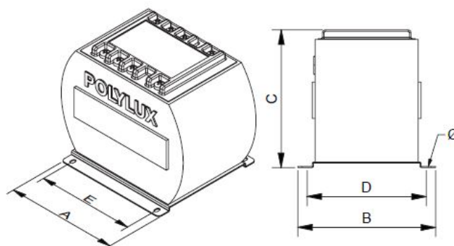
Dimensiones (AxBxCxDxE): 170x165x138x145x125 mm 7 
