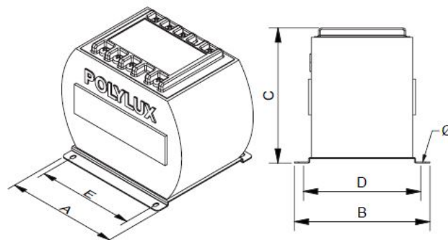
Dimensiones (AxBxCxDxE): 210x198x185x178x173 mm 7 
