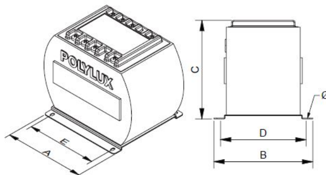
Dimensiones (AxBxCxDxE): 210x198x185x178x173 mm 7 
