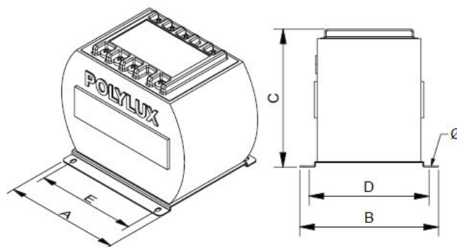
Dimensiones (AxBxCxDxE): 210x198x185x178x173 mm 7Ø
