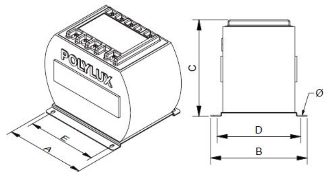
Dimensiones (AxBxCxDxE): 210x198x185x178x173 mm 7Ø
