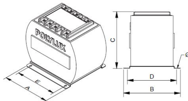
Dimensions (AxBxCxDxE): 135x145x108x125x102 mm 7Ø
