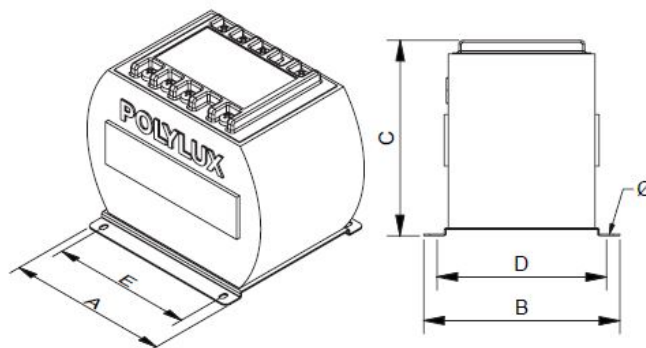
Dimensiones (Ax BxCxDxE): 135x145x108x125x102 mm 7Ø
