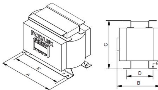
Dimensions (AxBxCxDxE): 280x190x205x115x250 mm 90°
