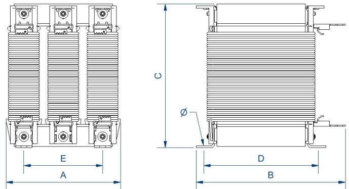
Dimensions (AxBxCxDxE): 150x145x185x84x100 mm 6Ø
