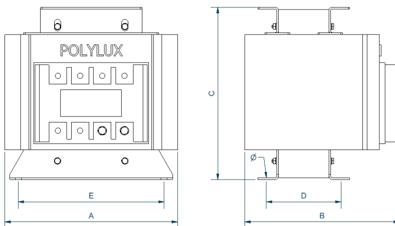
Dimensions (AxBxCxDxE): 280x202x419x142x210 mm 11Ø
