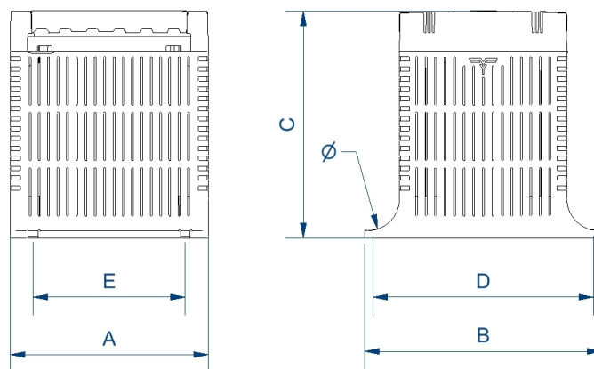
Dimensiones (AxBxCxDxE): 106x123x118x110x74 mm 5Ø
